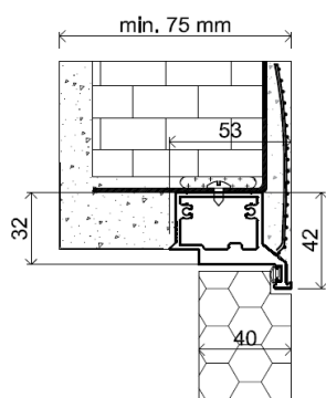
Standarta izmēri uz iekšu atveramām durvīm
